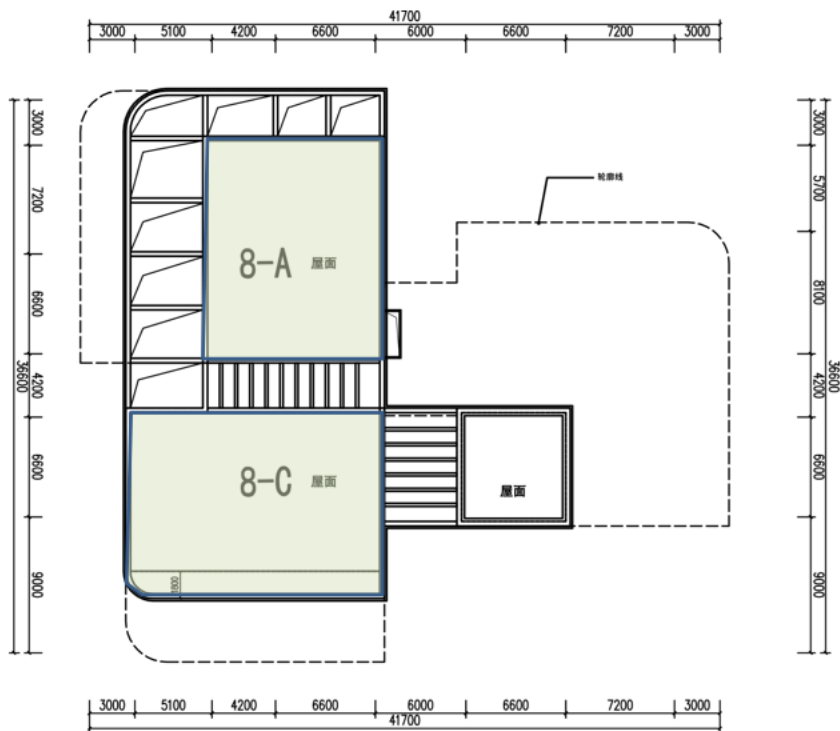
8/9号楼屋面层
